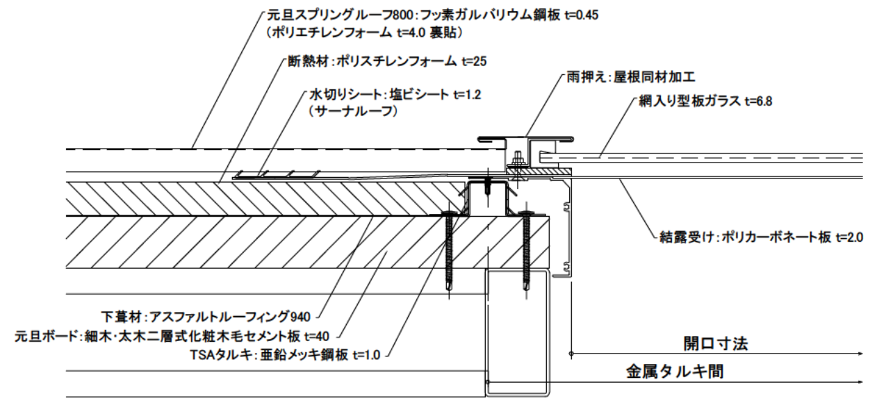
桁行方向断面図
