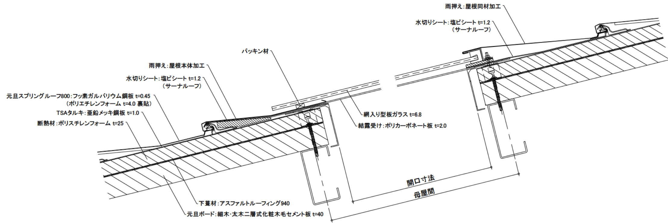
流れ方向断面図
