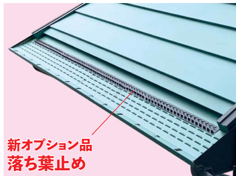
雪に強く落ち葉が入らない雨とい 元旦内樋
