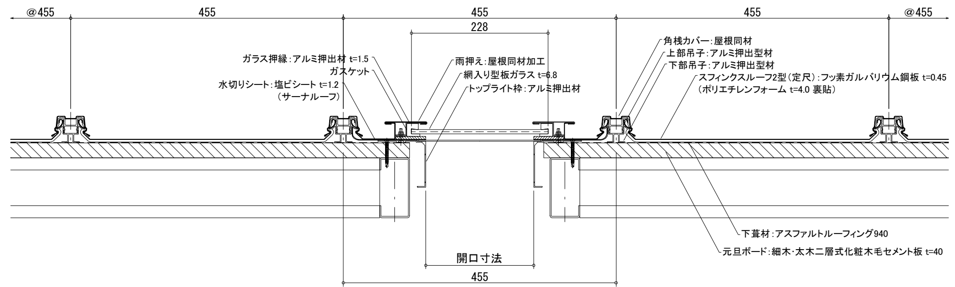
桁行方向断面図
